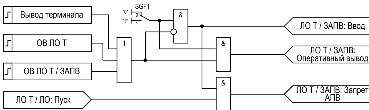
Рисунок 2.27 – Функциональная схема «ЗАПВ»
