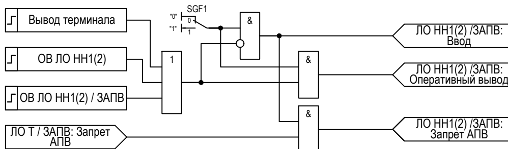
Рисунок 2.30 – Функциональная схема «Запрет АПВ»
