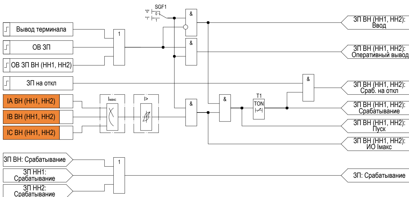
Рисунок 2.13 – Функциональная схема «ЗП»
