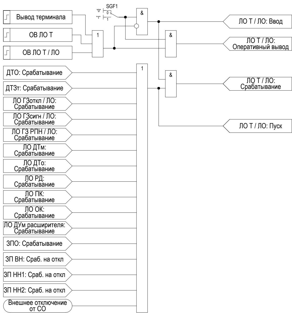
Рисунок 2.26 – Функциональная схема «ЛО»
