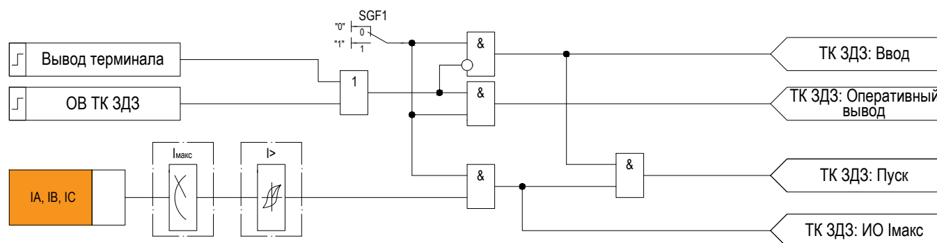
Рисунок 2.15 – Функциональная схема «ТК ЗДЗ»
