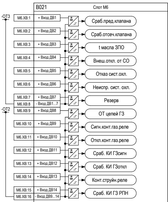
Рисунок И.3 – Подключение дискретных входов и выходов к внутренним сигналам алгоритмов для плат в слотах М5-М7
