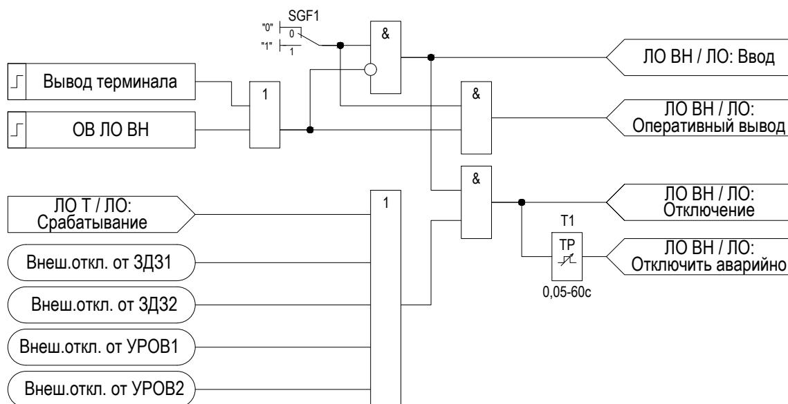
Рисунок 2.28 – Функциональная схема «ЛО»
