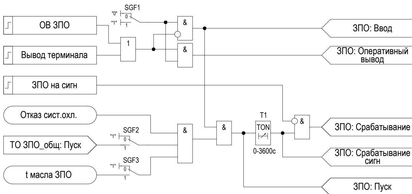
Рисунок 2.11 – Функциональная схема «ЗПО»
