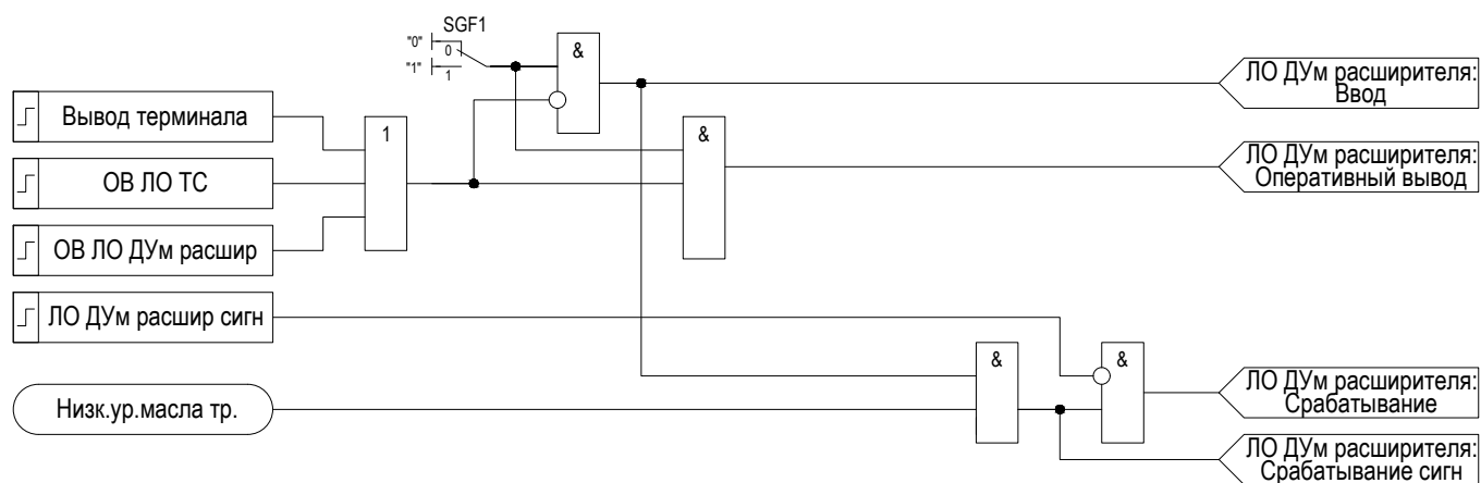
Рисунок 2.25 – Функциональная схема «ЛО ДУм расширителя»
