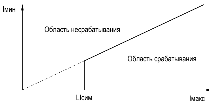
Рисунок 2.10 – Характеристика срабатывания функции контроля токовых цепей стороны трансформатора
