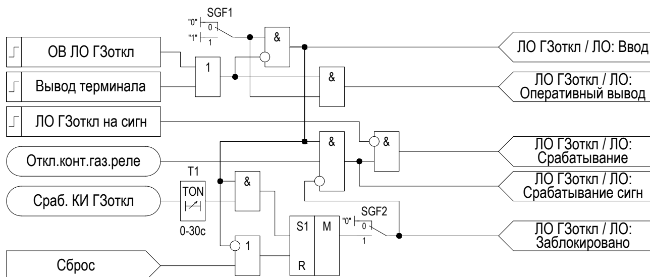
Рисунок 2.17 – Функциональная схема «ЛО ГЗоткл»
