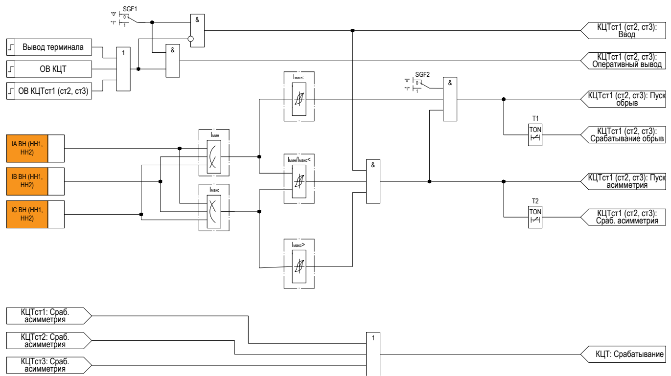
Рисунок 2.9 – Функциональная схема «КЦТ»
