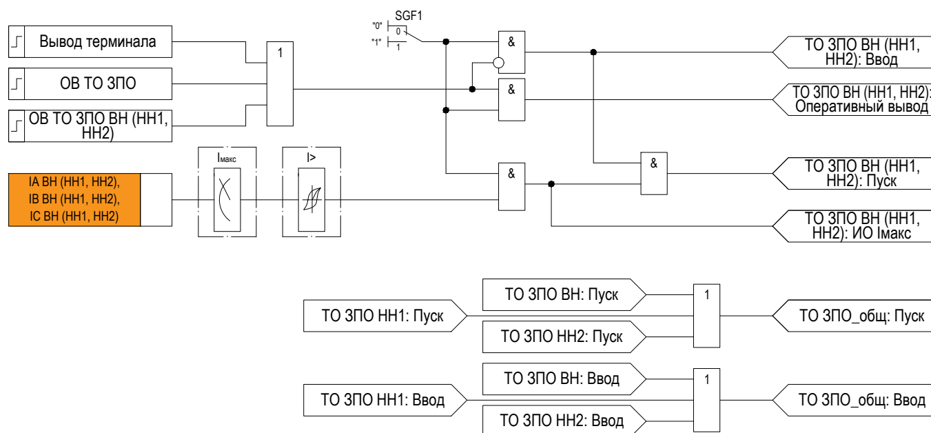
Рисунок 2.12 – Функциональная схема «ТО ЗПО»
