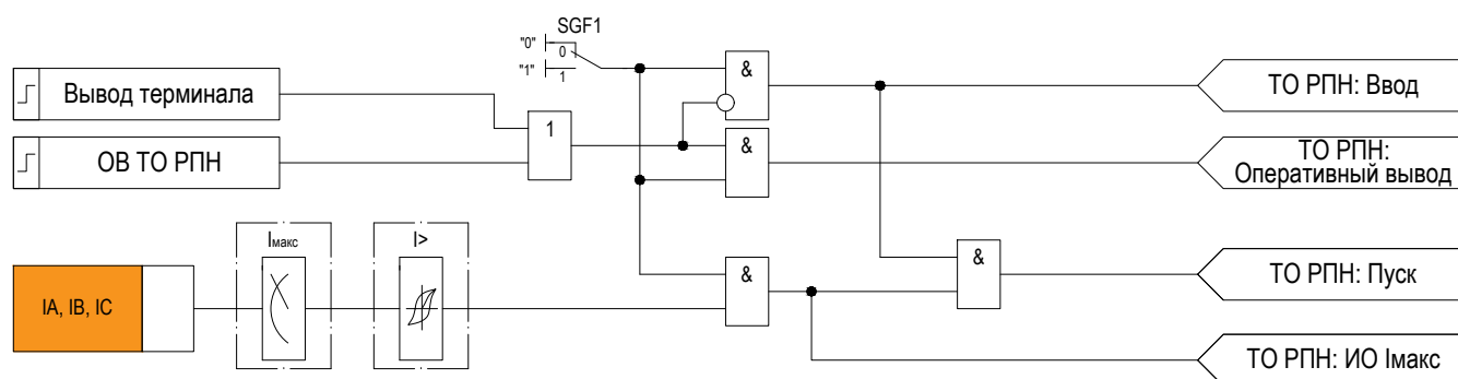
Рисунок 2.16 – Функциональная схема «ТО РПН»
