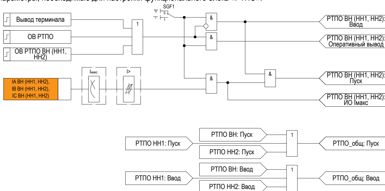
Рисунок 2.14 – Функциональная схема «РТПО»
