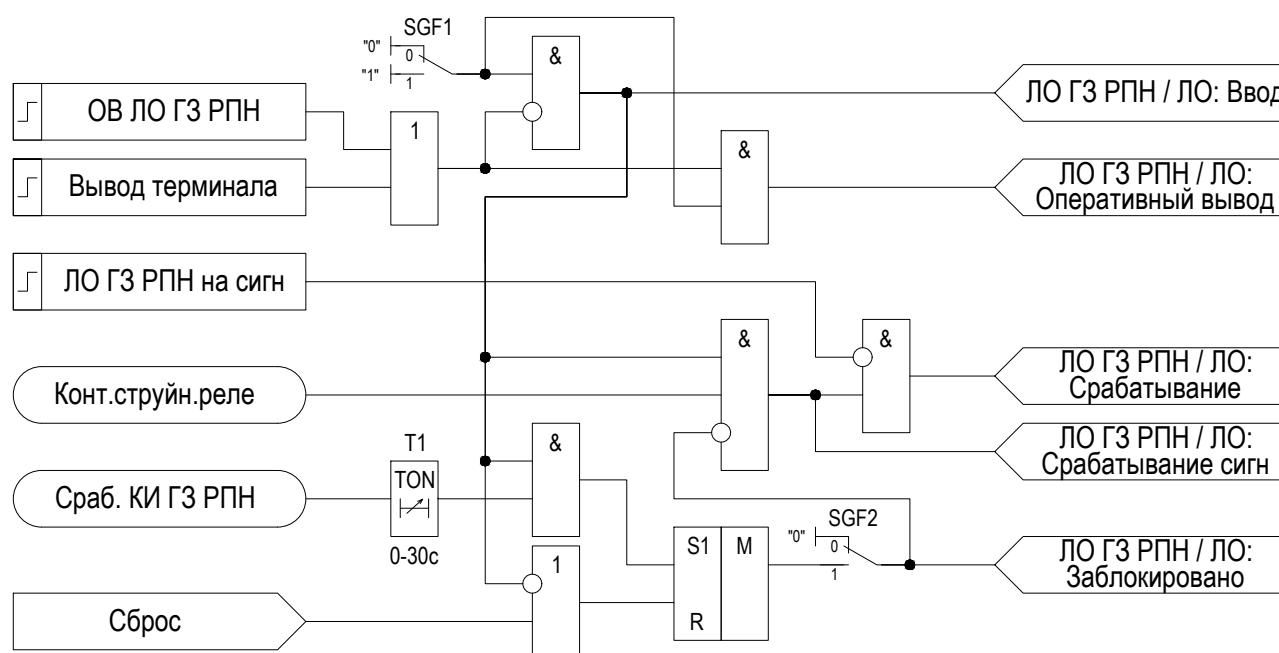
Рисунок 2.19 – Функциональная схема «ЛО ГЗ РПН»
