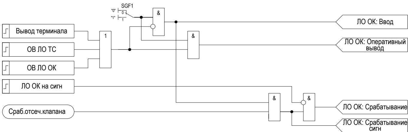
Рисунок 2.24 – Функциональная схема «ЛО ОК»
