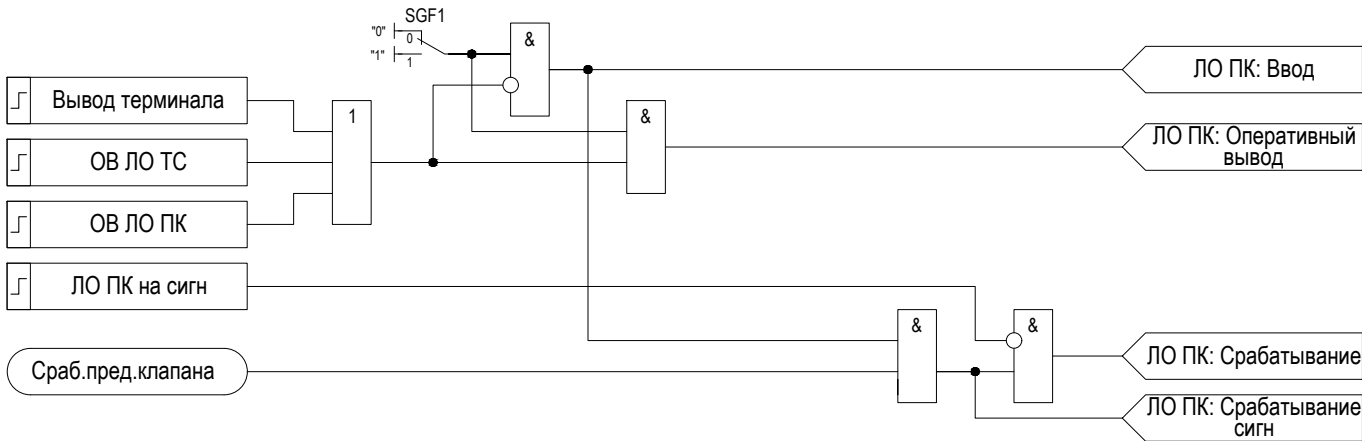
Рисунок 2.23 – Функциональная схема «ЛО ПК»
