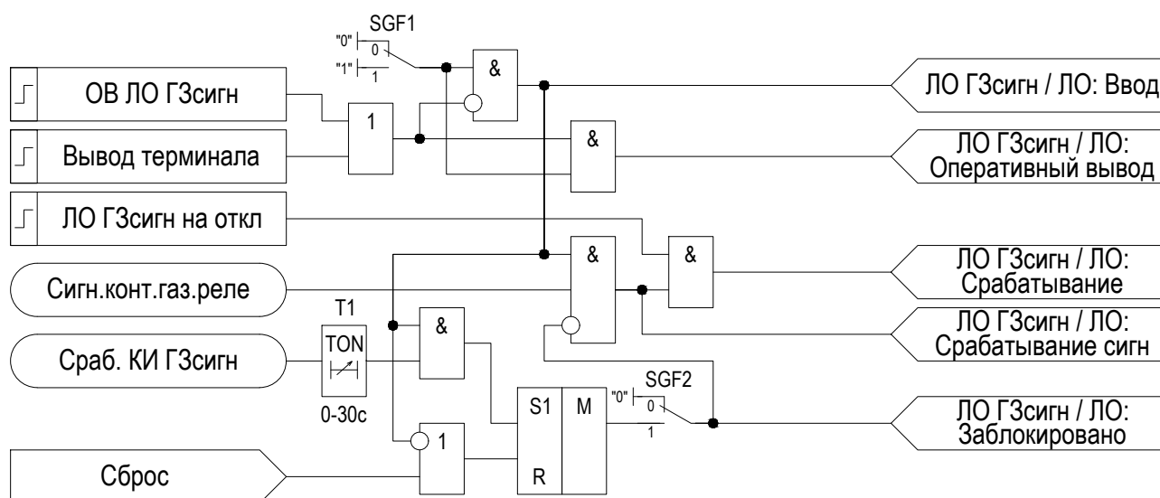
Рисунок 2.18 – Функциональная схема «ЛО ГЗсигн»
